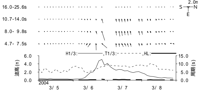
図 - 11.26 むつ小川原 周期帯別波浪特性の経時変化(高波期間中)
