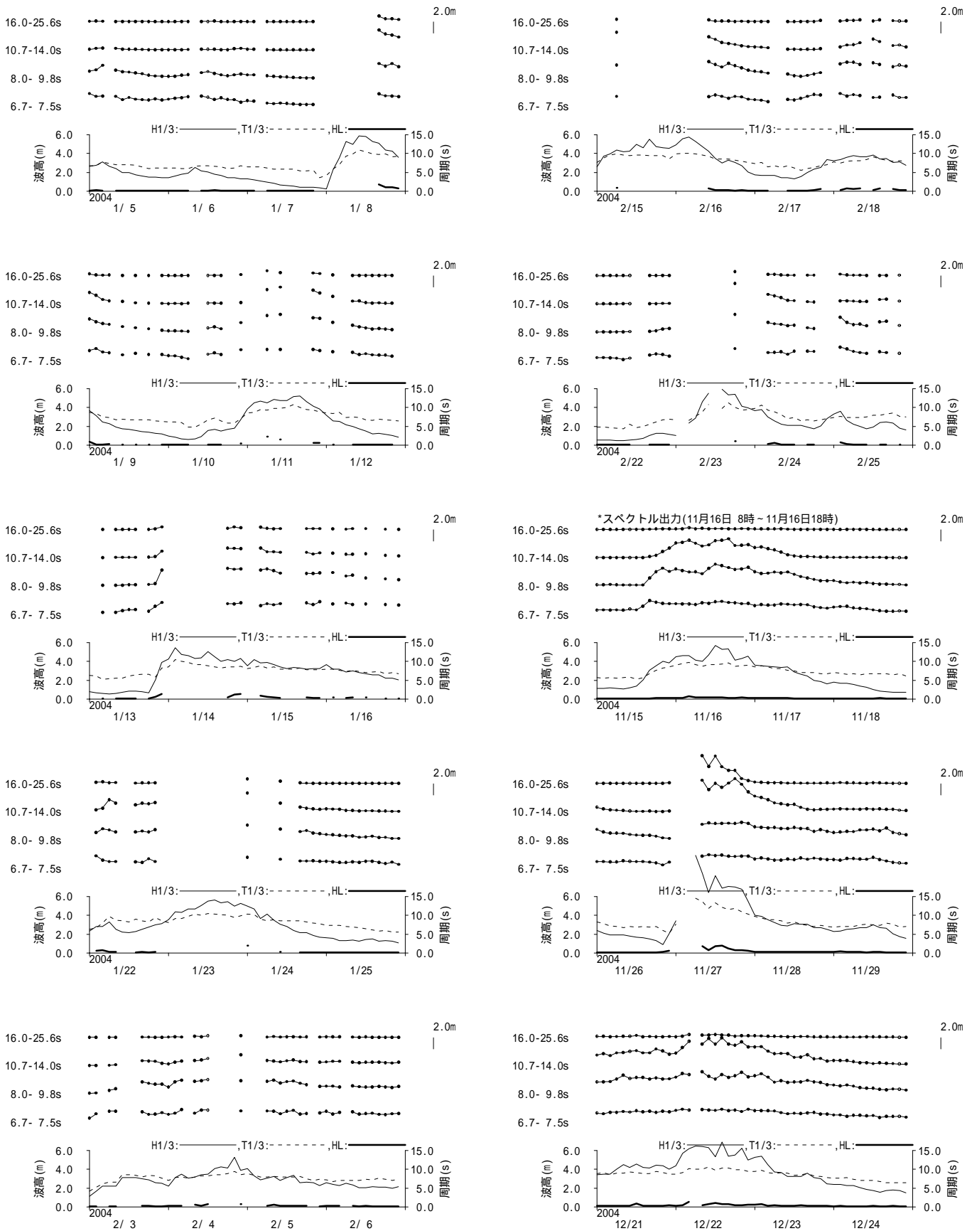
図 - 11.4 深浦 周期帯別波浪特性の経時変化(高波期間中)
