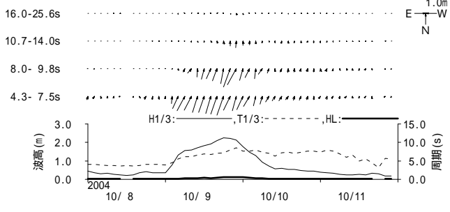
図 - 11.9 富山 周期帯別波浪特性の経時変化(高波期間中)
