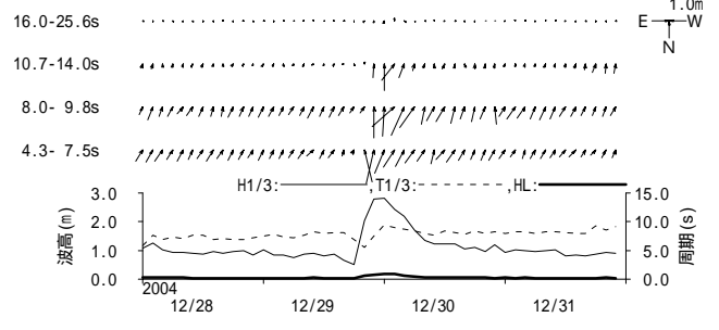
図 - 11.9 富山 周期帯別波浪特性の経時変化(高波期間中)
