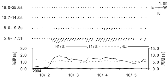
図 - 11.10 伏木富山 周期帯別波浪特性の経時変化(高波期間中)
