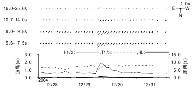
図 - 11.10 伏木富山 周期帯別波浪特性の経時変化(高波期間中)
