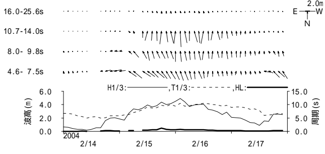
図 - 11.7 新潟沖 周期帯別波浪特性の経時変化(高波期間中)
