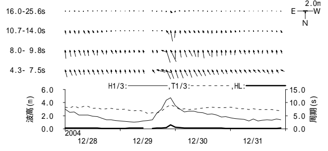
図 - 11.12 金沢 周期帯別波浪特性の経時変化(高波期間中)
