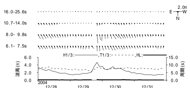
図 - 11.11 輪島 周期帯別波浪特性の経時変化(高波期間中)
