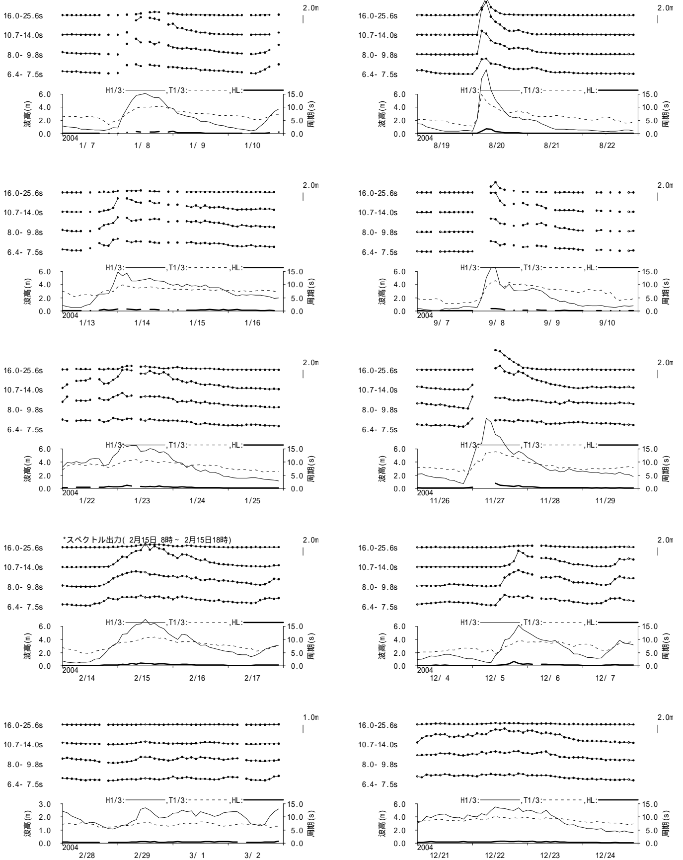
図 - 11.6 酒田 周期帯別波浪特性の経時変化(高波期間中)
