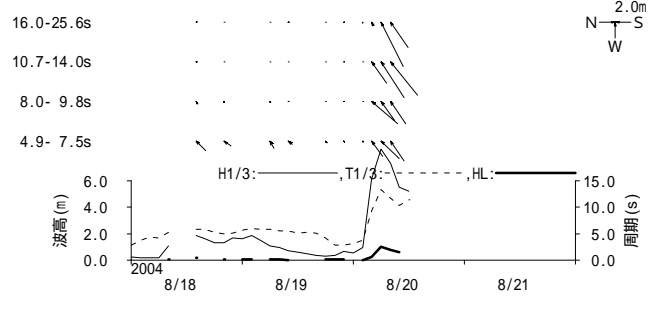
図 - 11.5 秋田 周期帯別波浪特性の経時変化(高波期間中)
