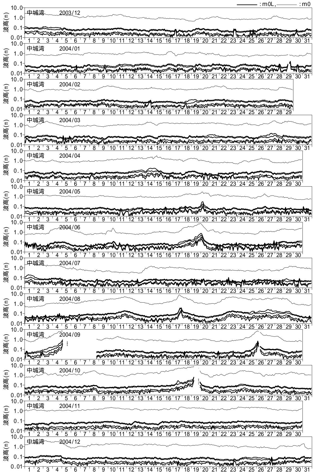
図 - 10.54 長周期波高の経時変化図 (中城湾)
