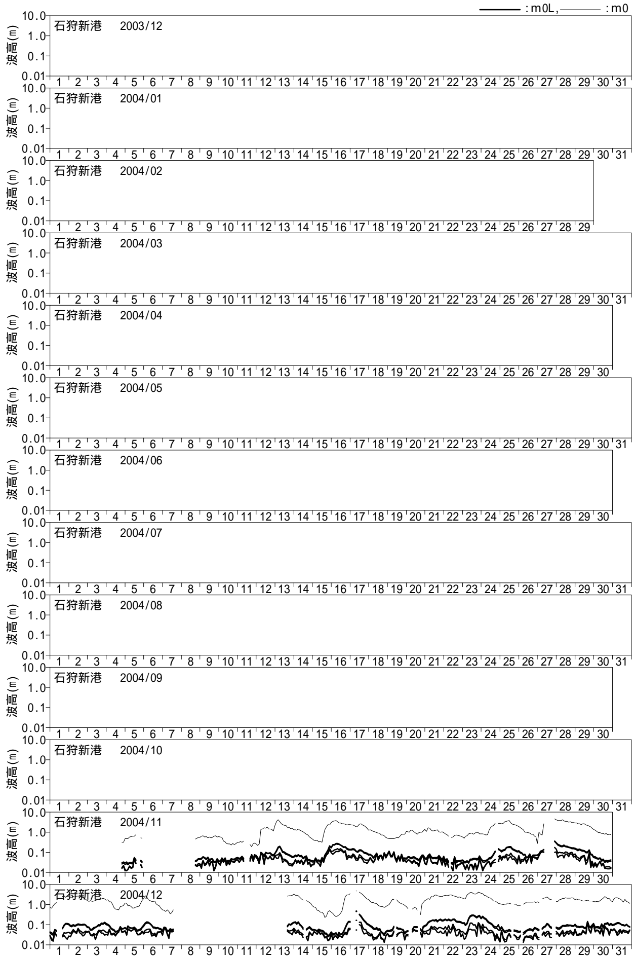
図 - 10.2 長周期波高の経時変化図 (石狩新港)
