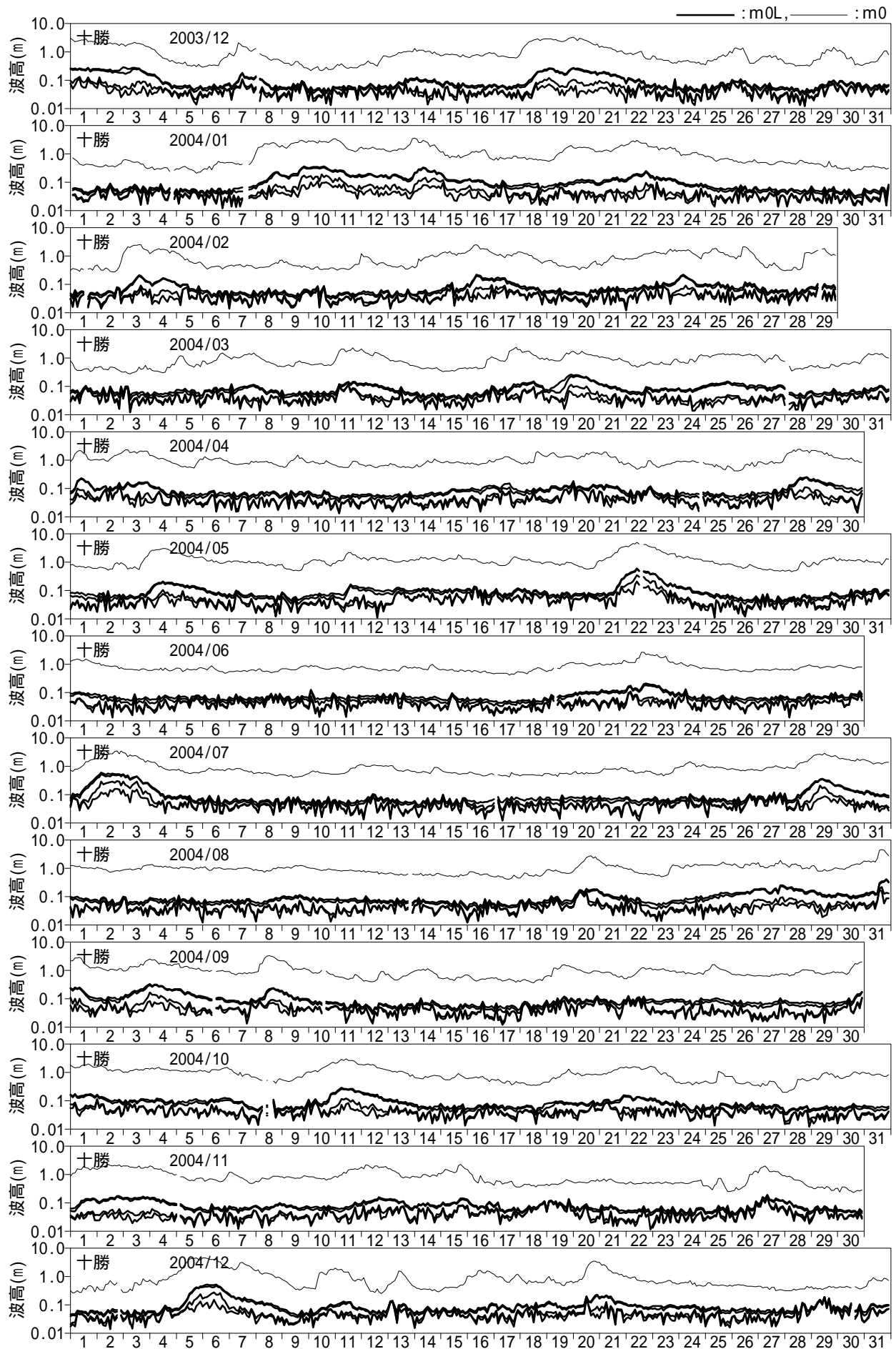
図 - 10.24 長周期波高の経時変化図 (十勝)
