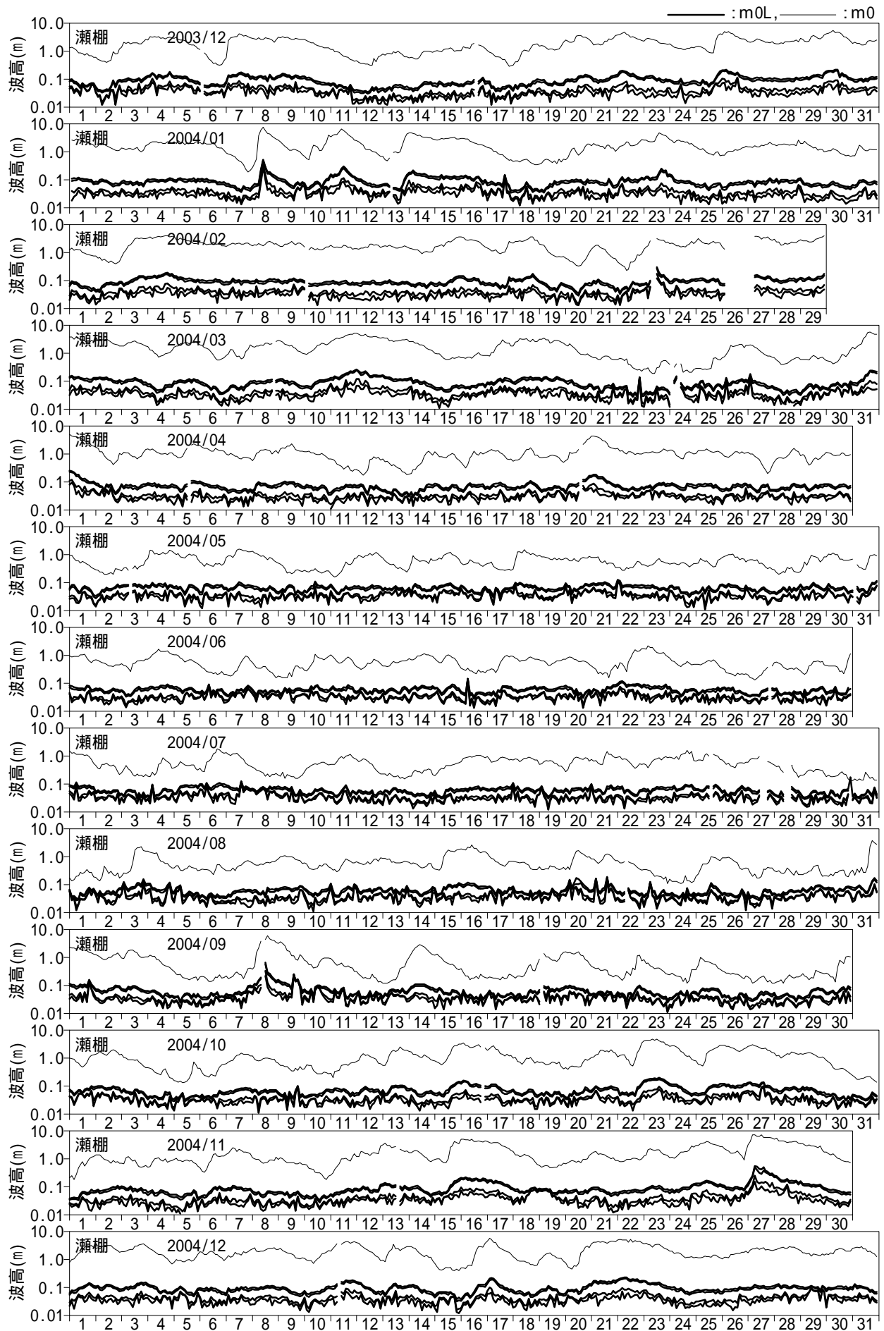
図 - 10.3 長周期波高の経時変化図 (瀬棚)
