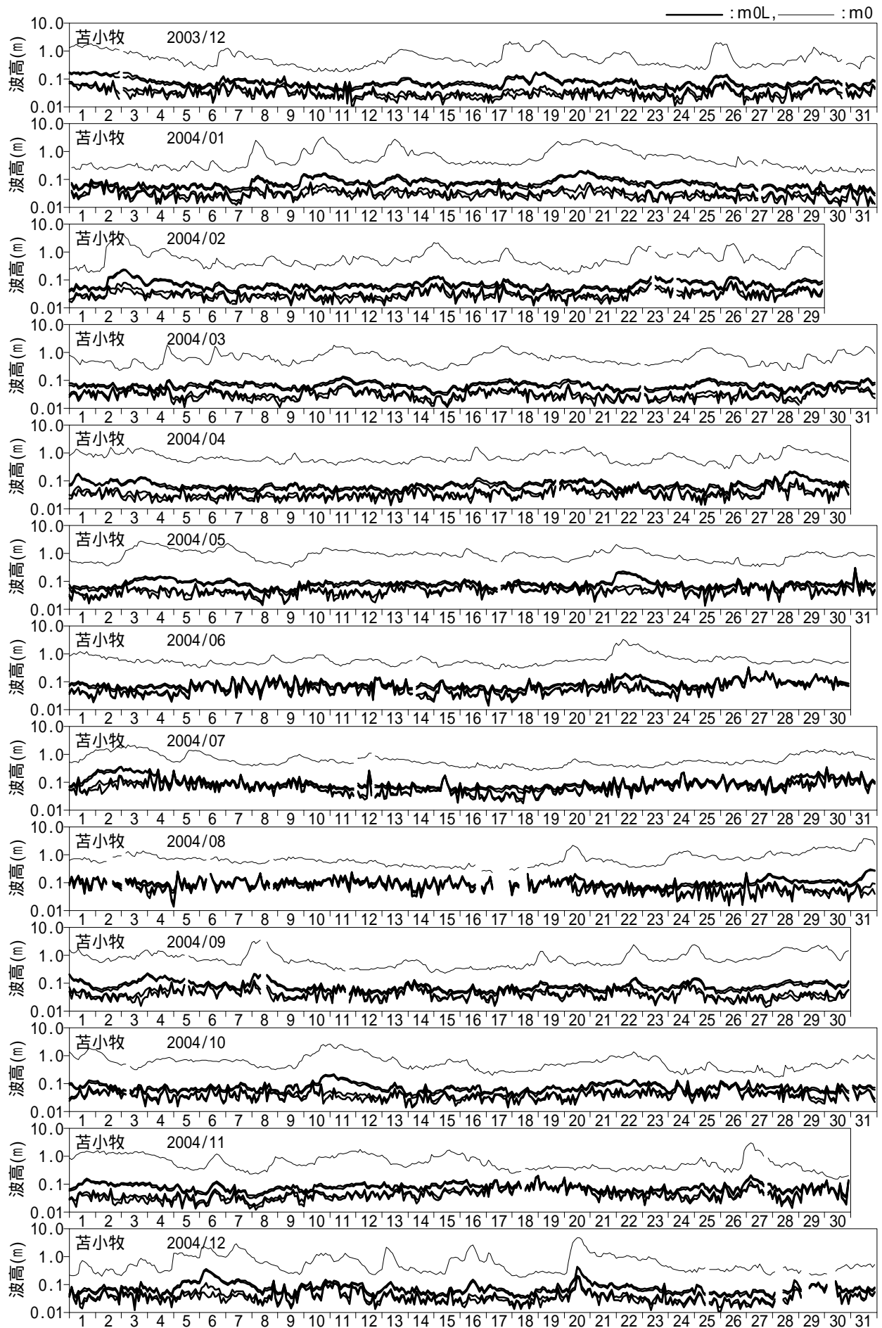
図 - 10.25 長周期波高の経時変化図 (苦小牧)
