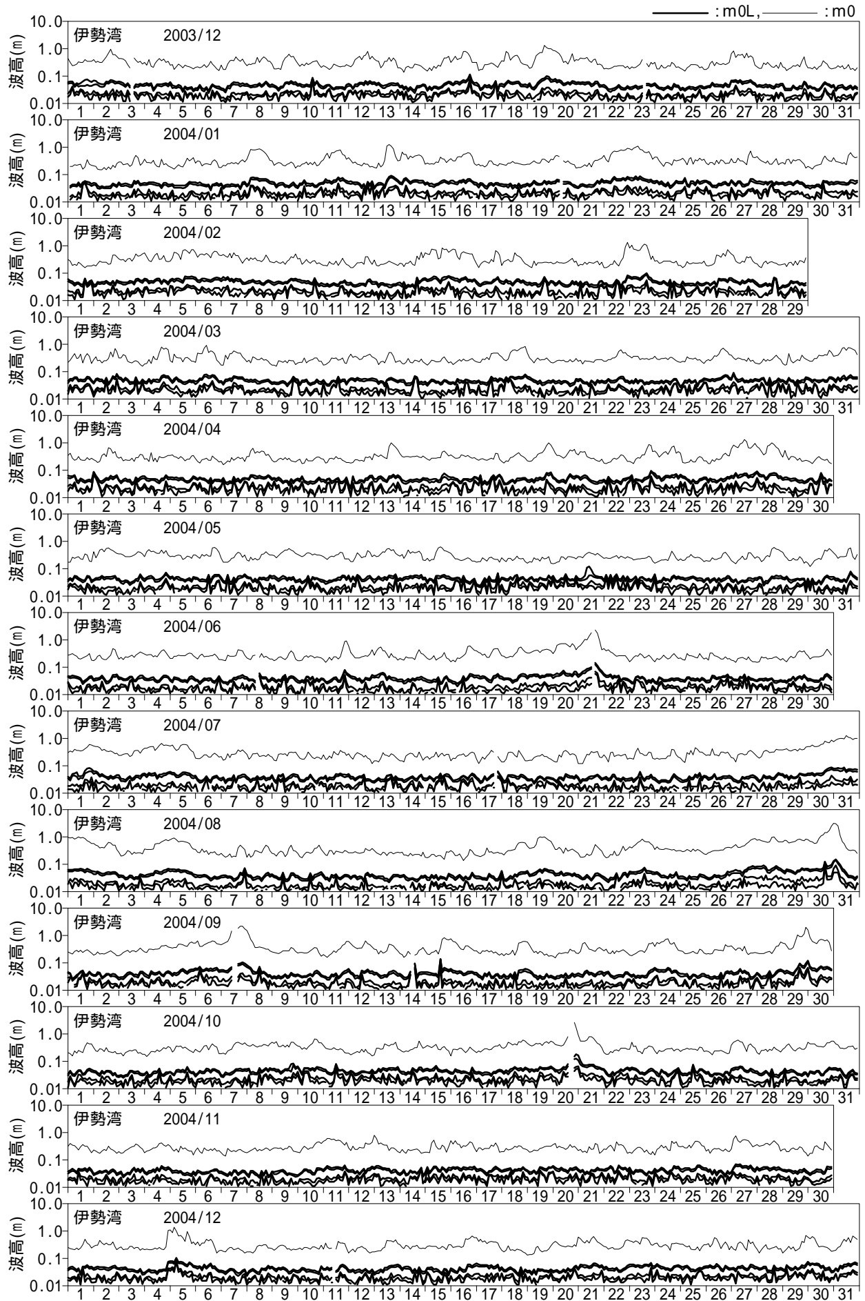
図 - 10.42 長周期波高の経時変化図 (伊勢湾)
