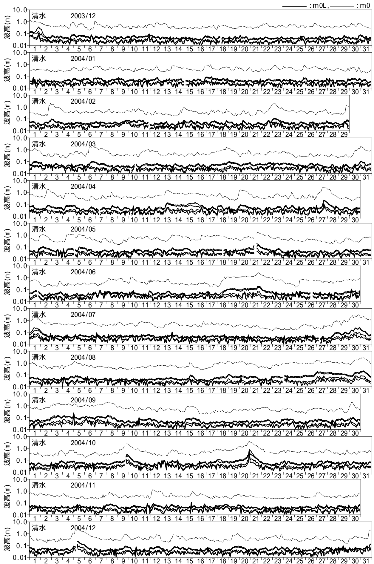
図 - 10.40 長周期波高の経時変化図 (清水)
