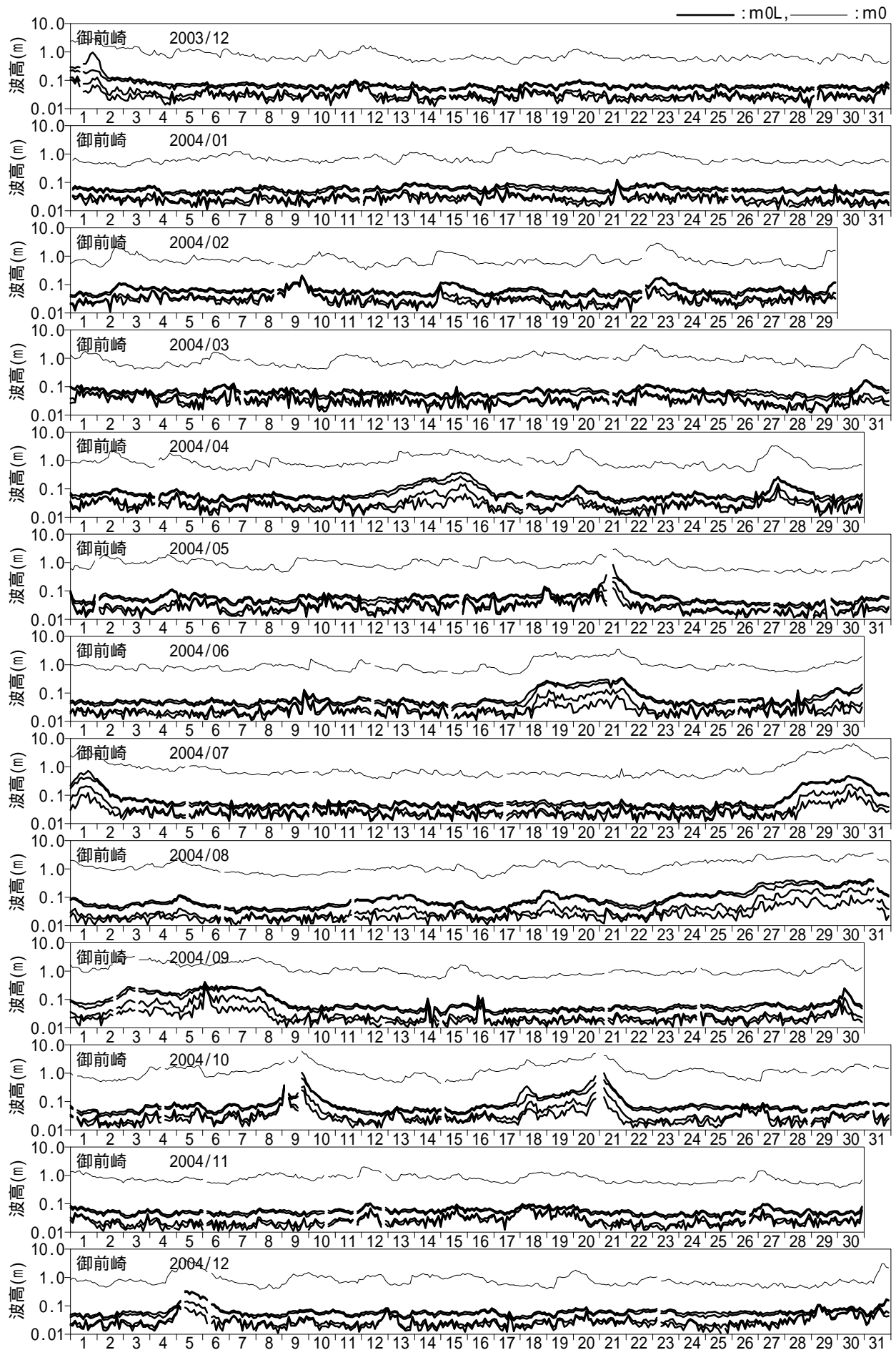
図 - 10.41 長周期波高の経時変化図 (御前崎)
