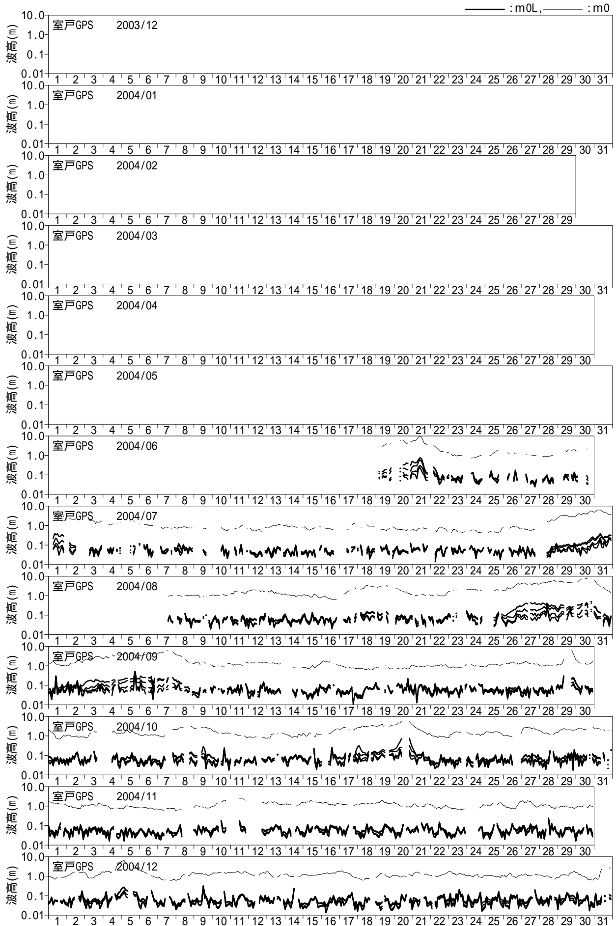
図 - 10.46 長周期波高の経時変化図 (室戸GPS)
