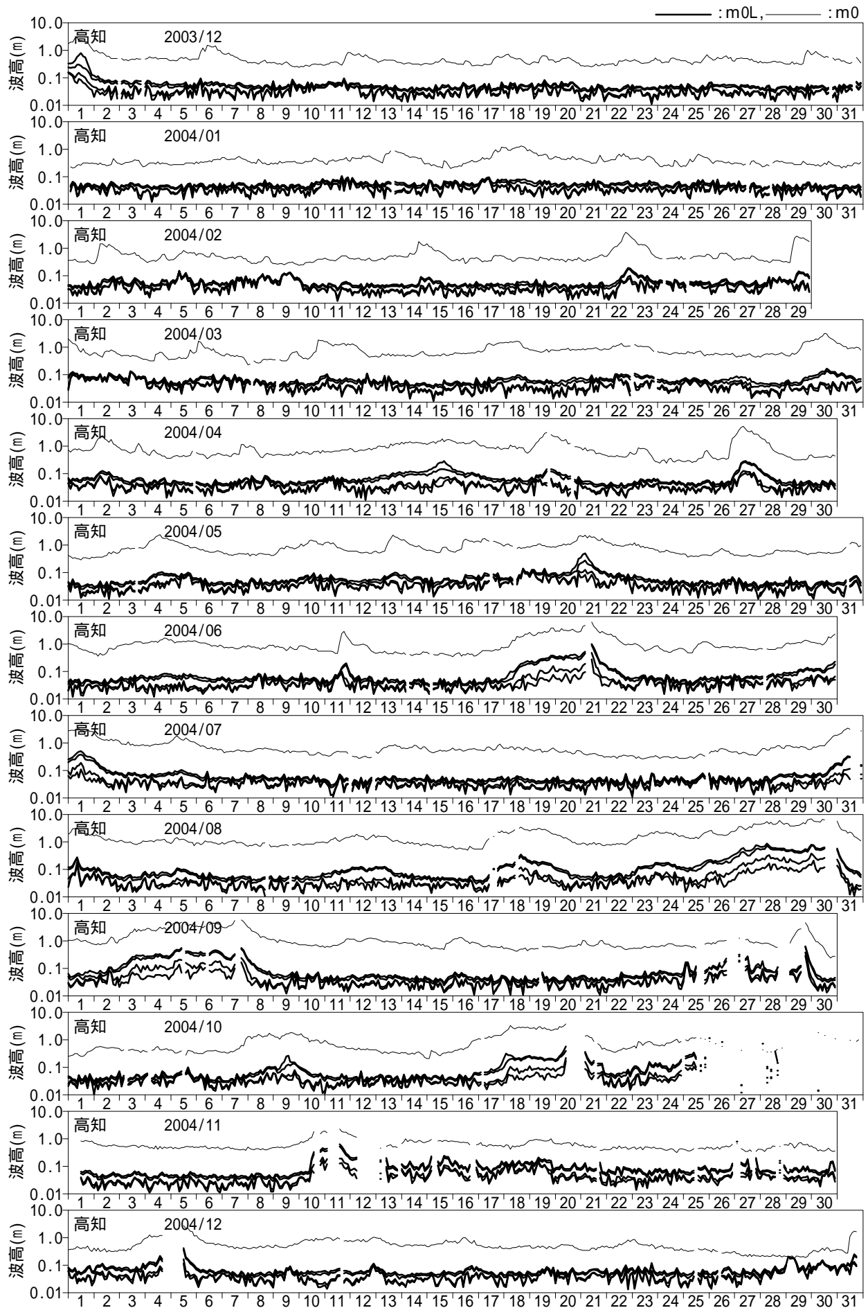
図 - 10.48 長周期波高の経時変化図 (高知)
