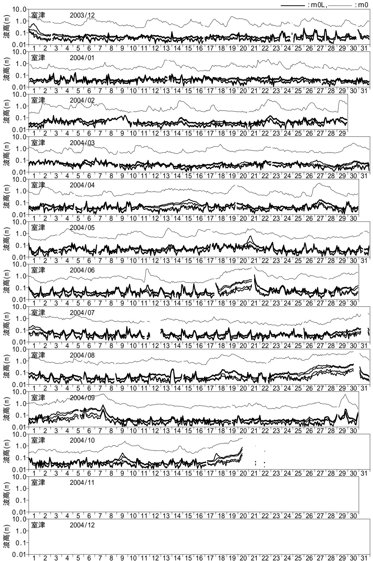
図 - 10.47 長周期波高の経時変化図 (室津)
