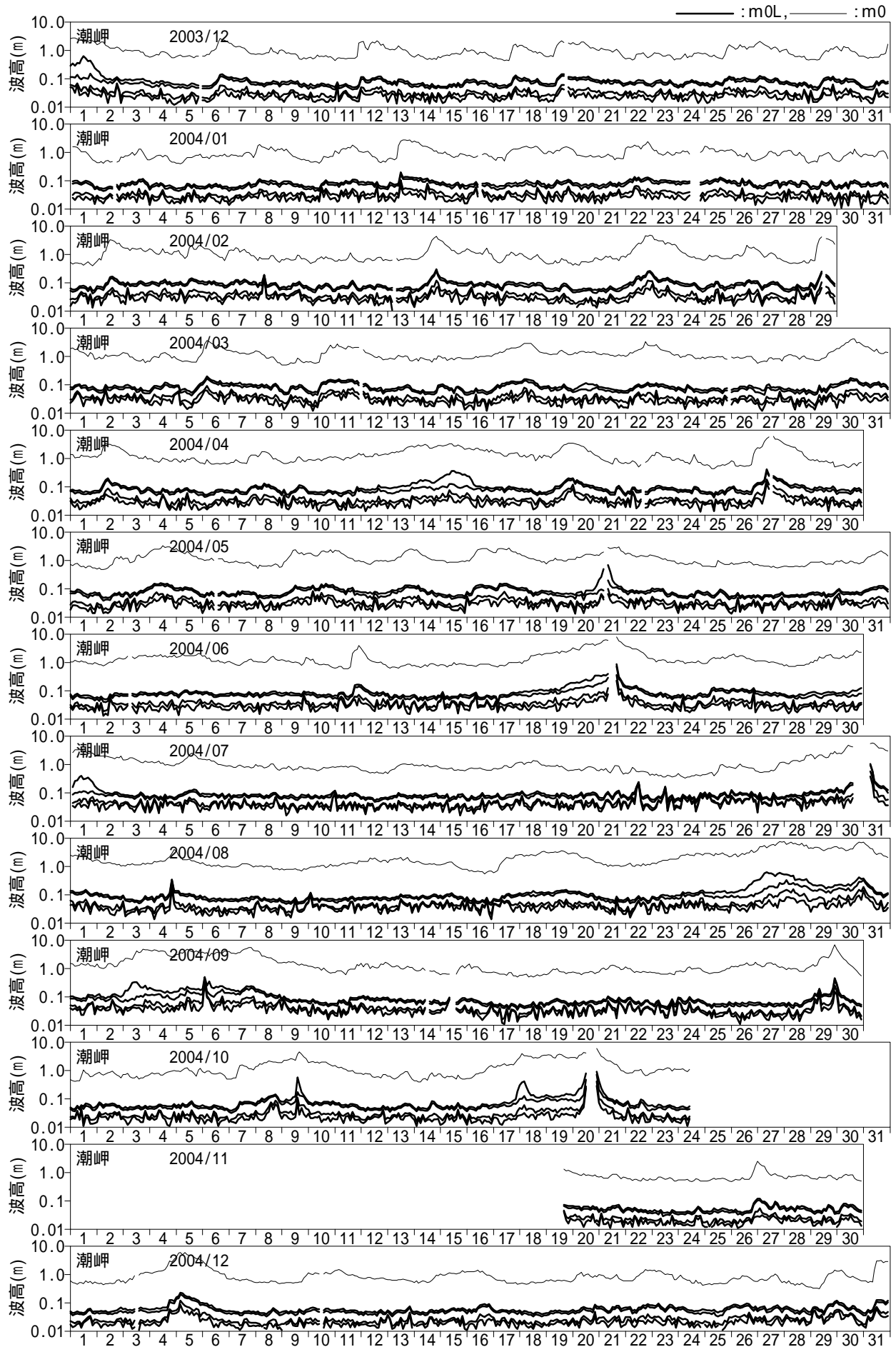
図 - 10.43 長周期波高の経時変化図 (潮岬)
