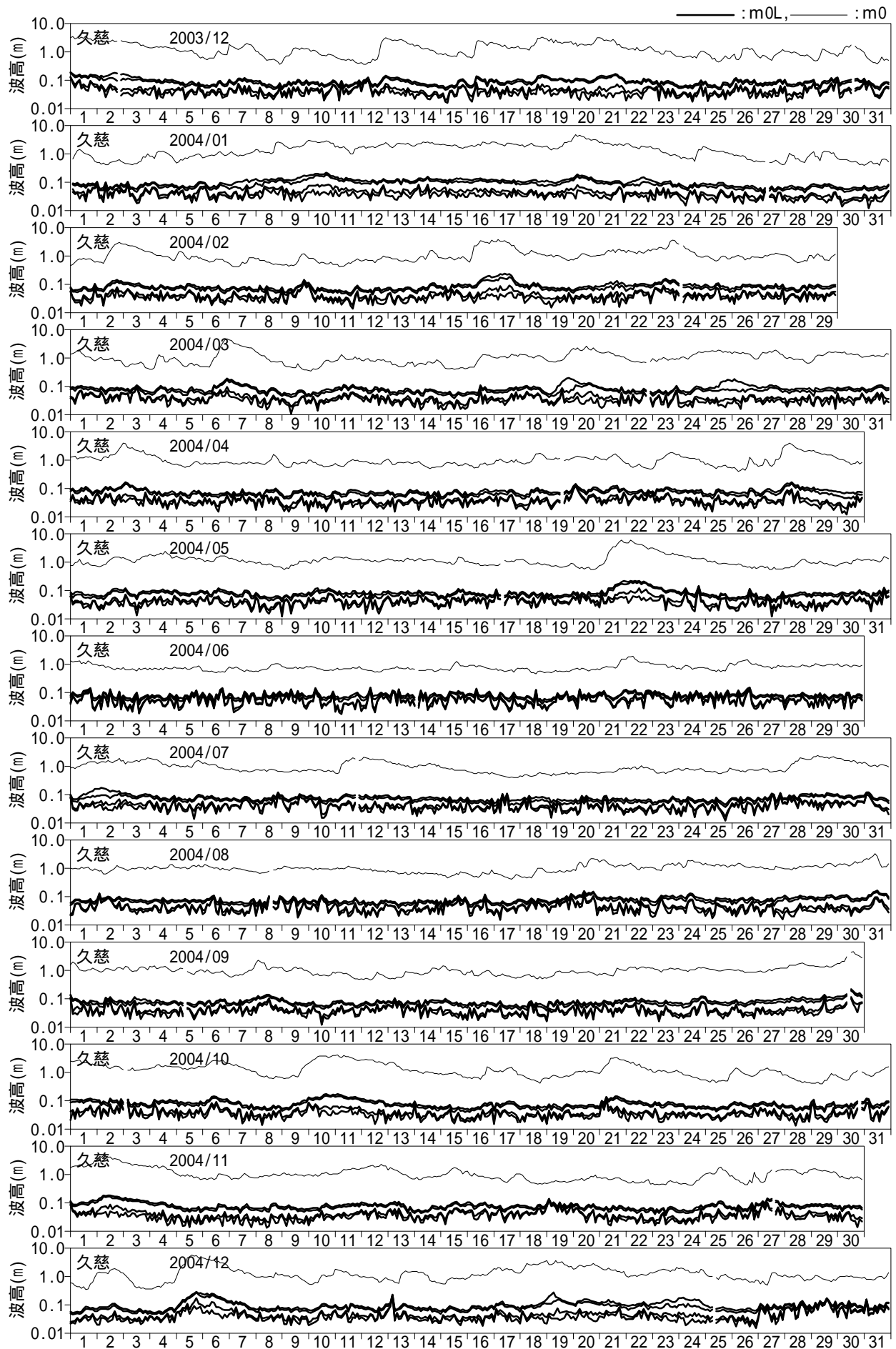
図 - 10.28 長周期波高の経時変化図(久慈)
