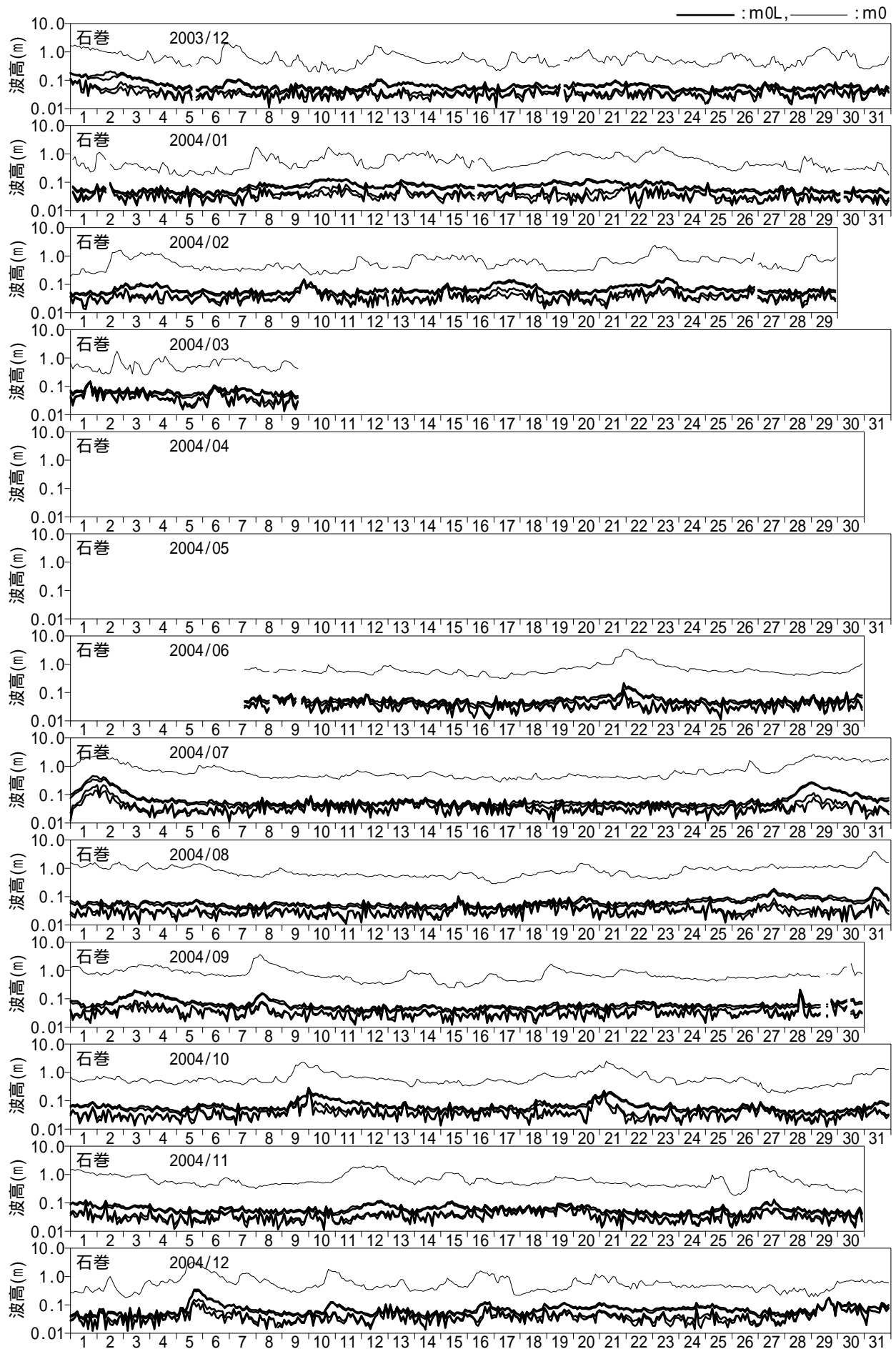
図 - 10.30 長周期波高の経時変化図 (石巻)
