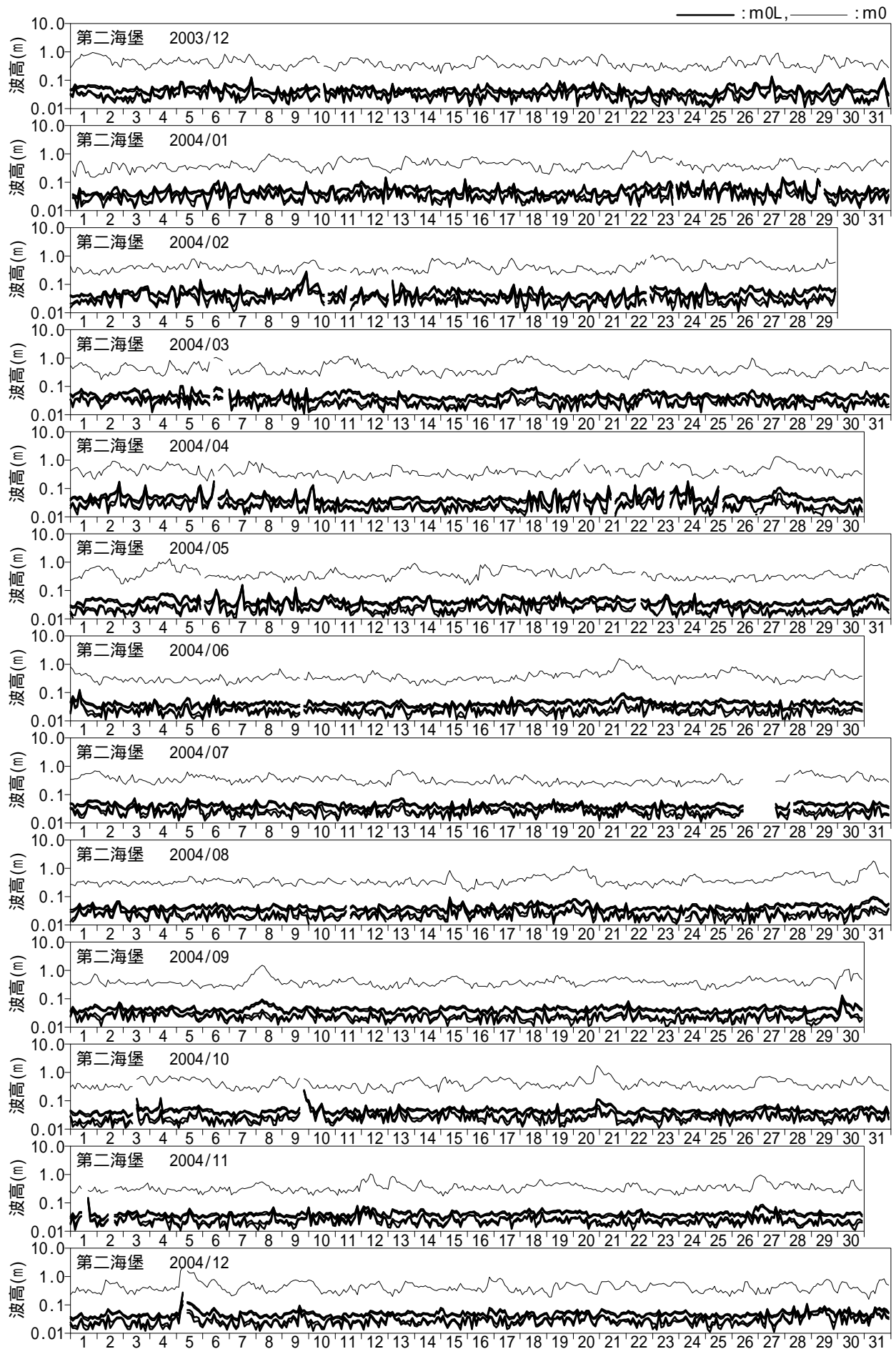
図 - 10.36 長周期波高の経時変化図 (第二海堡)
