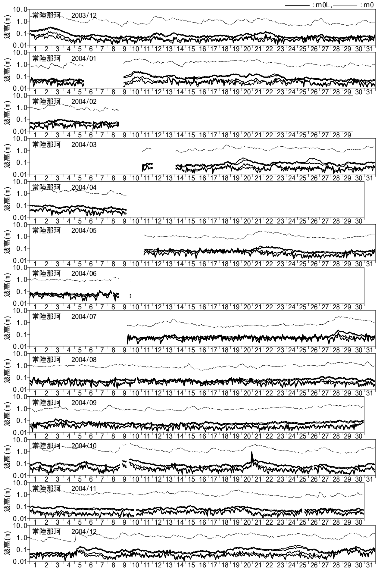
図 - 10.34 長周期波高の経時変化図 (常陸那珂)
