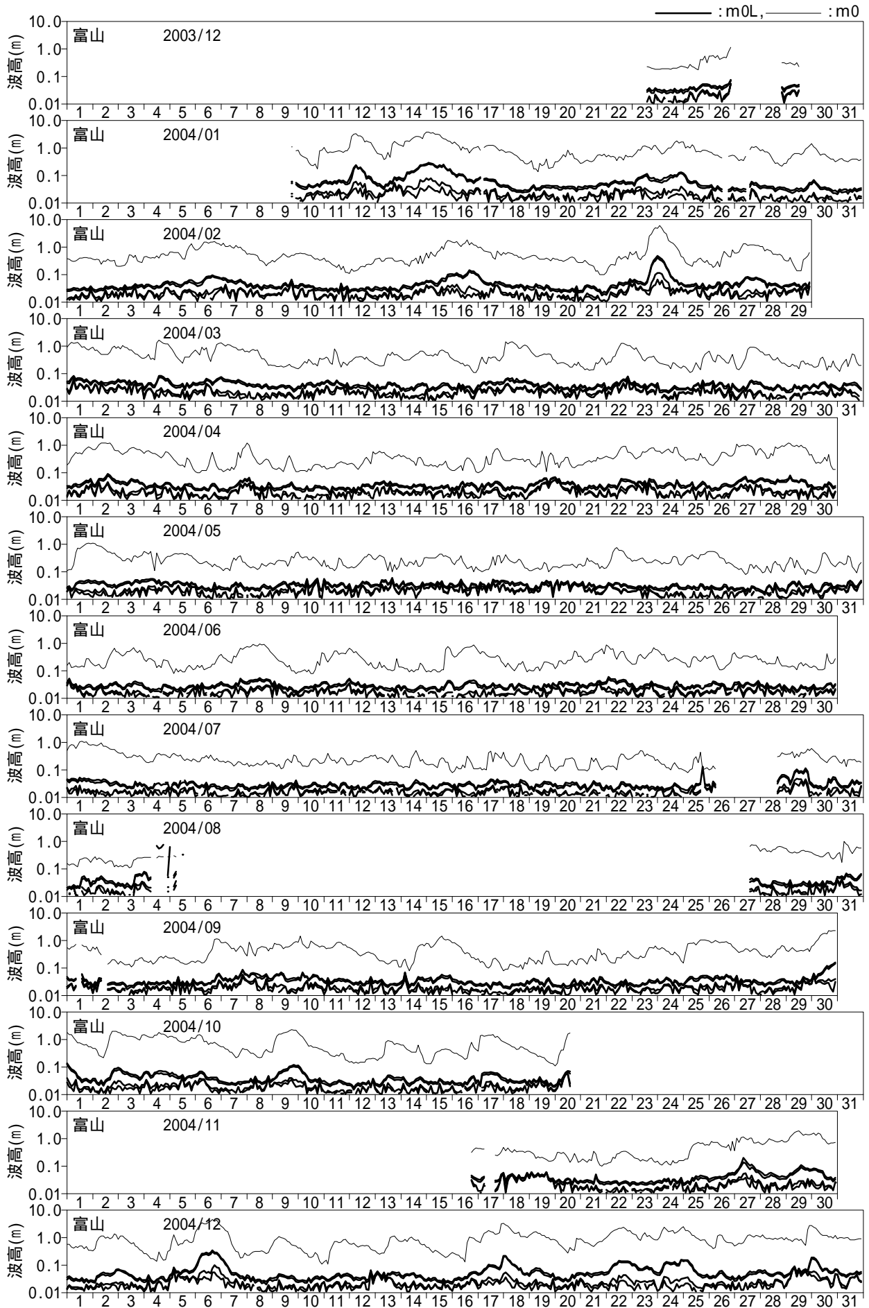
図 - 10.9 長周期波高の経時変化図 (富山)
