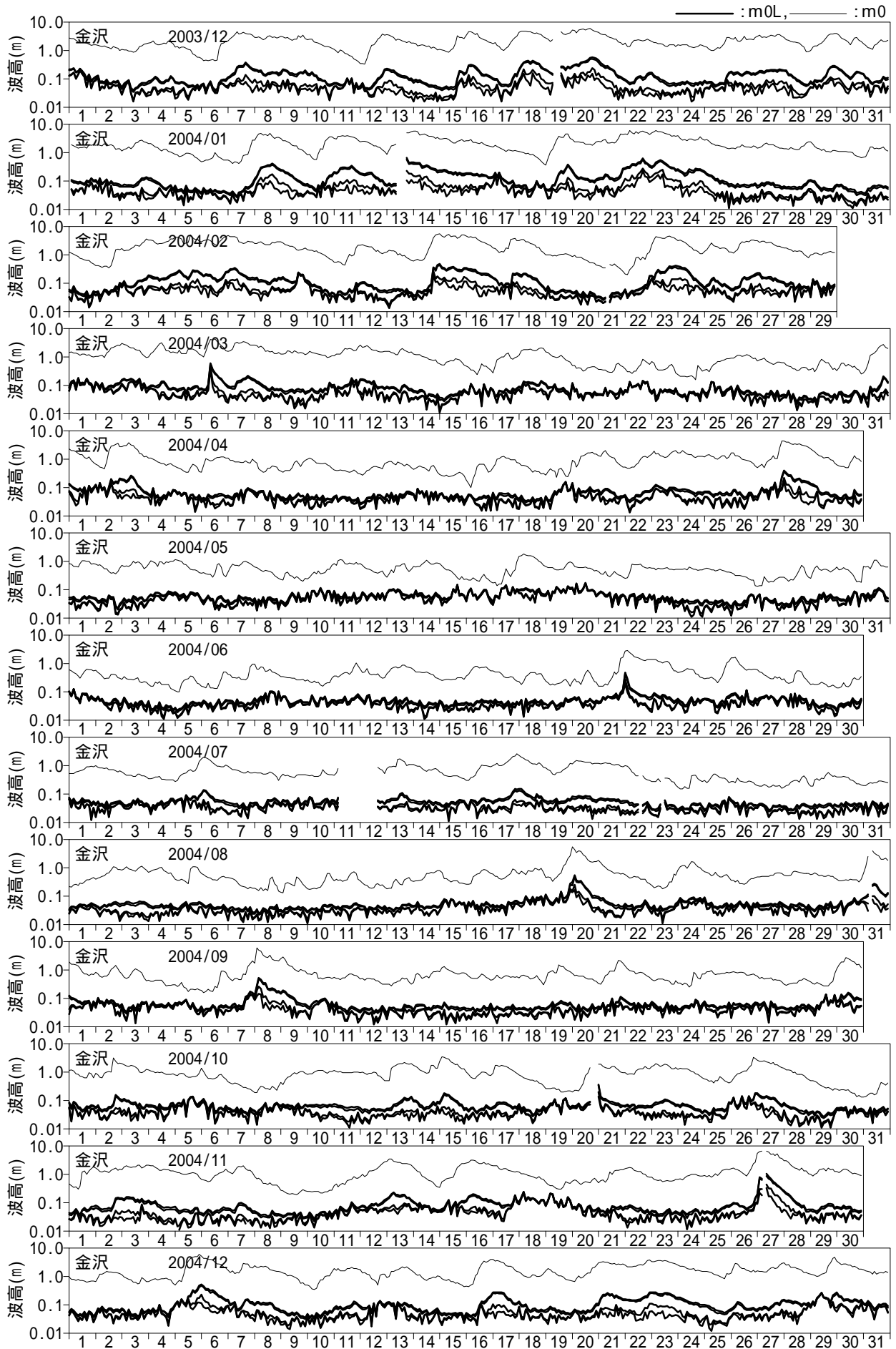
図 - 10.12 長周期波高の経時変化図 (金沢)
