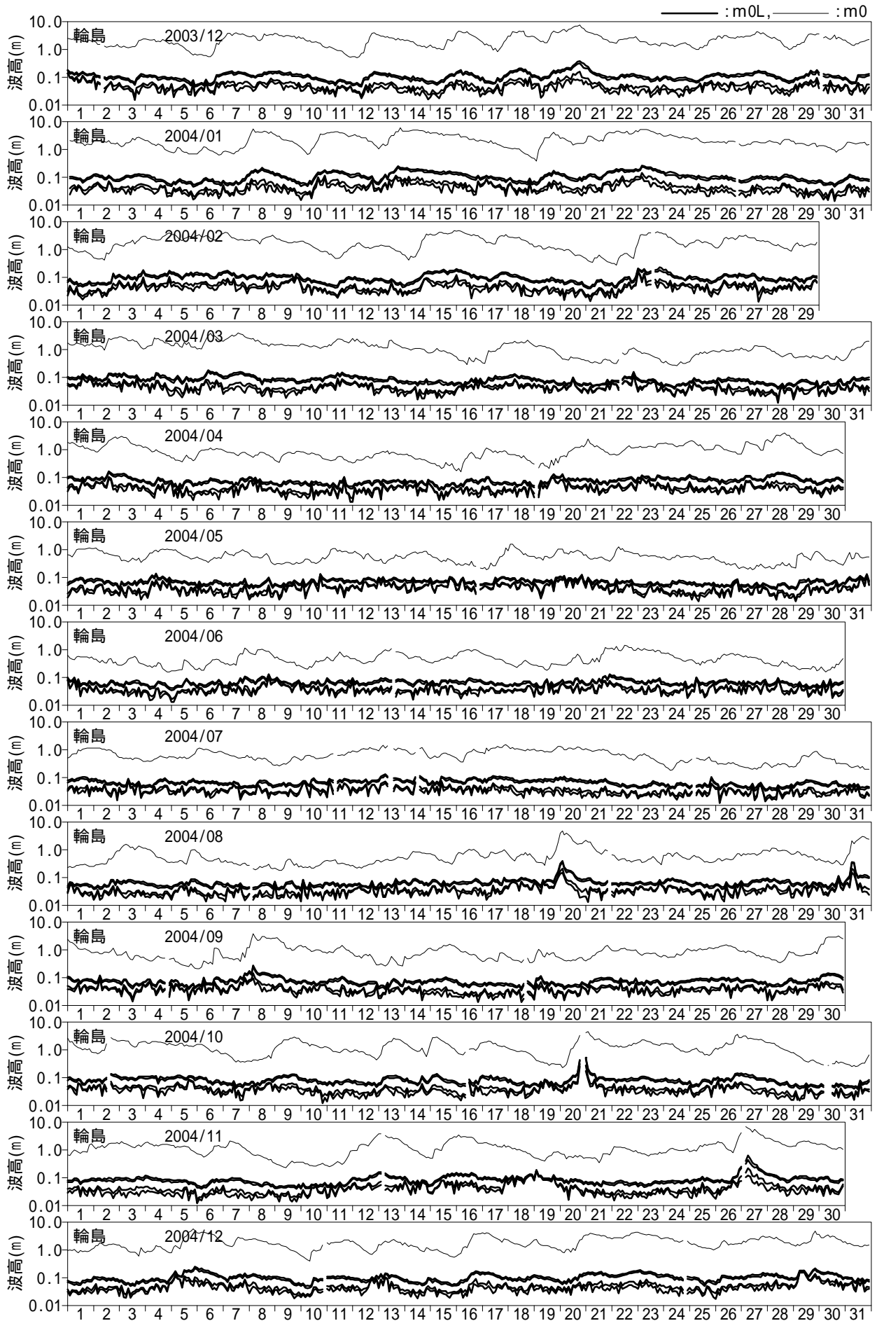
図 - 10.11 長周期波高の経時変化図 (輪島)
