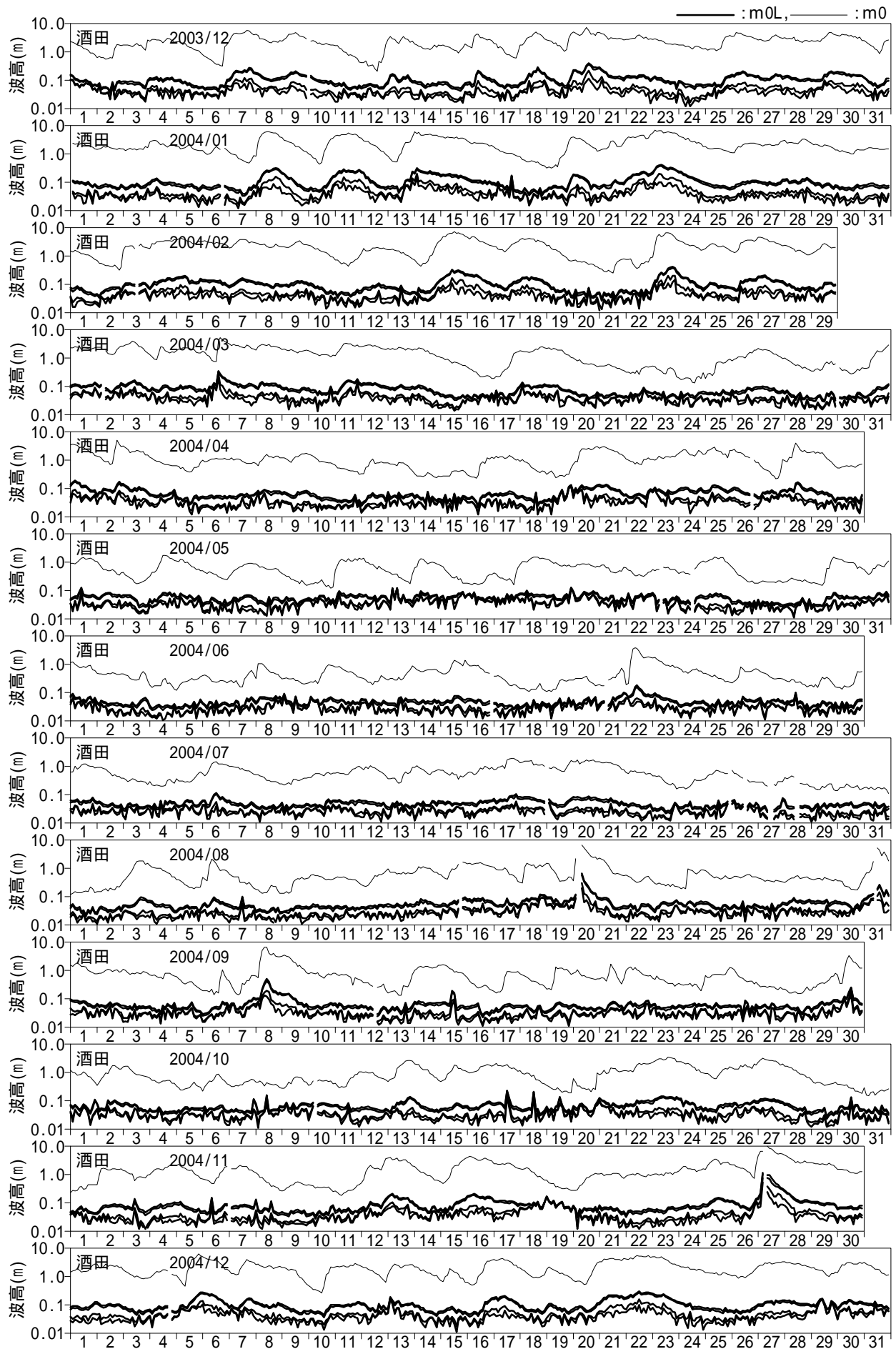
図 - 10.6 長周期波高の経時変化図 (酒田)
