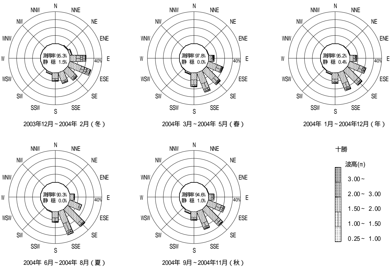
図 - 8.24 十勝 波高・波向別出現頻度図
