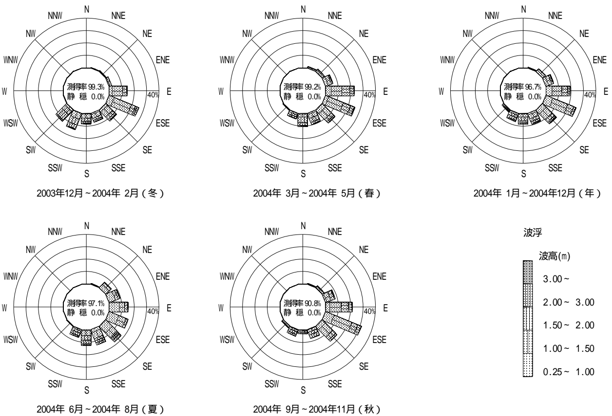
図 - 8.38 波浮 波高・波向別出現頻度図
