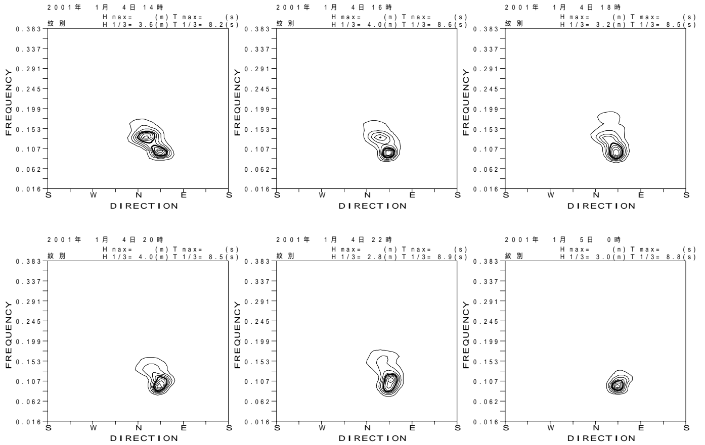
付図 - B.3.21 紋別 代表的な高波期間中の方向スペクトル
