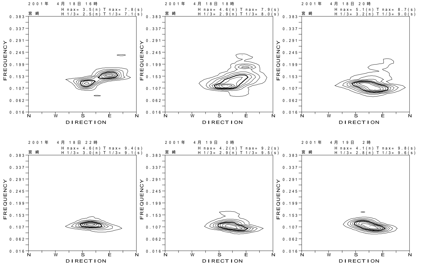
付図 - B.3.47 宮崎 代表的な高波期間中の方向スペクトル
