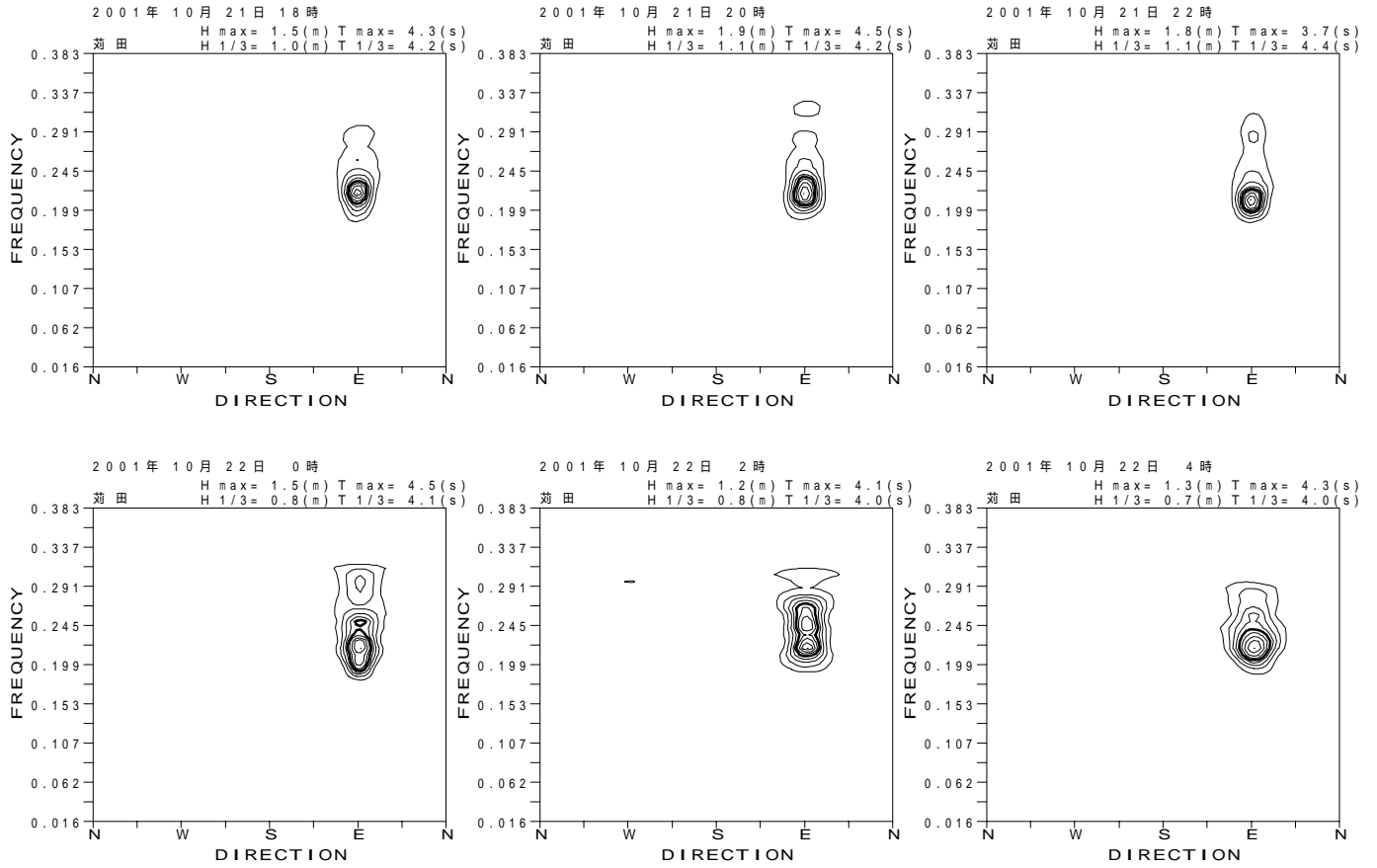
付図 - B.3.46 荻田 代表的な高波期間中の方向スペクトル
