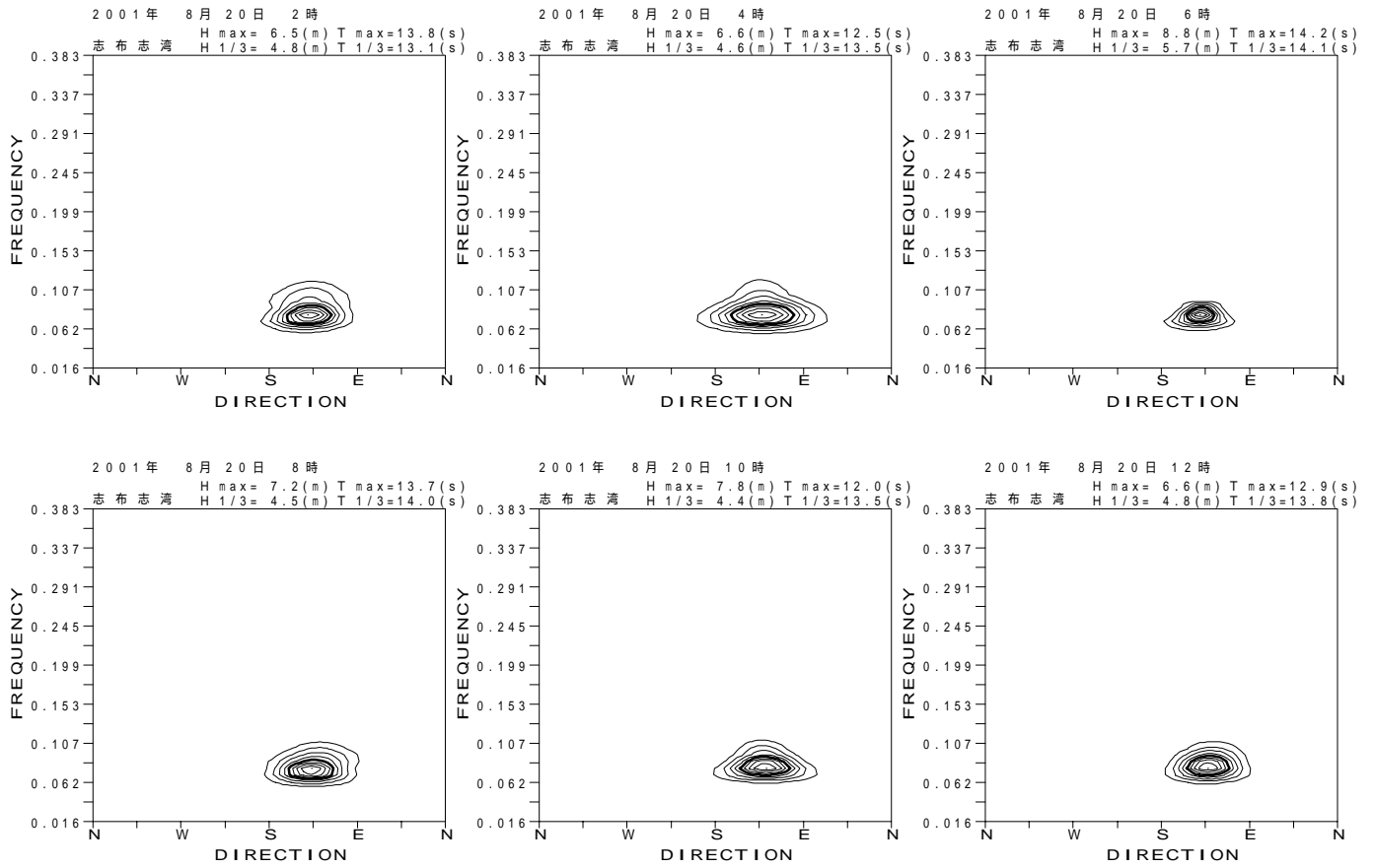
付図 - B.3.48 志布志湾 代表的な高波期間中の方向スペクトル
