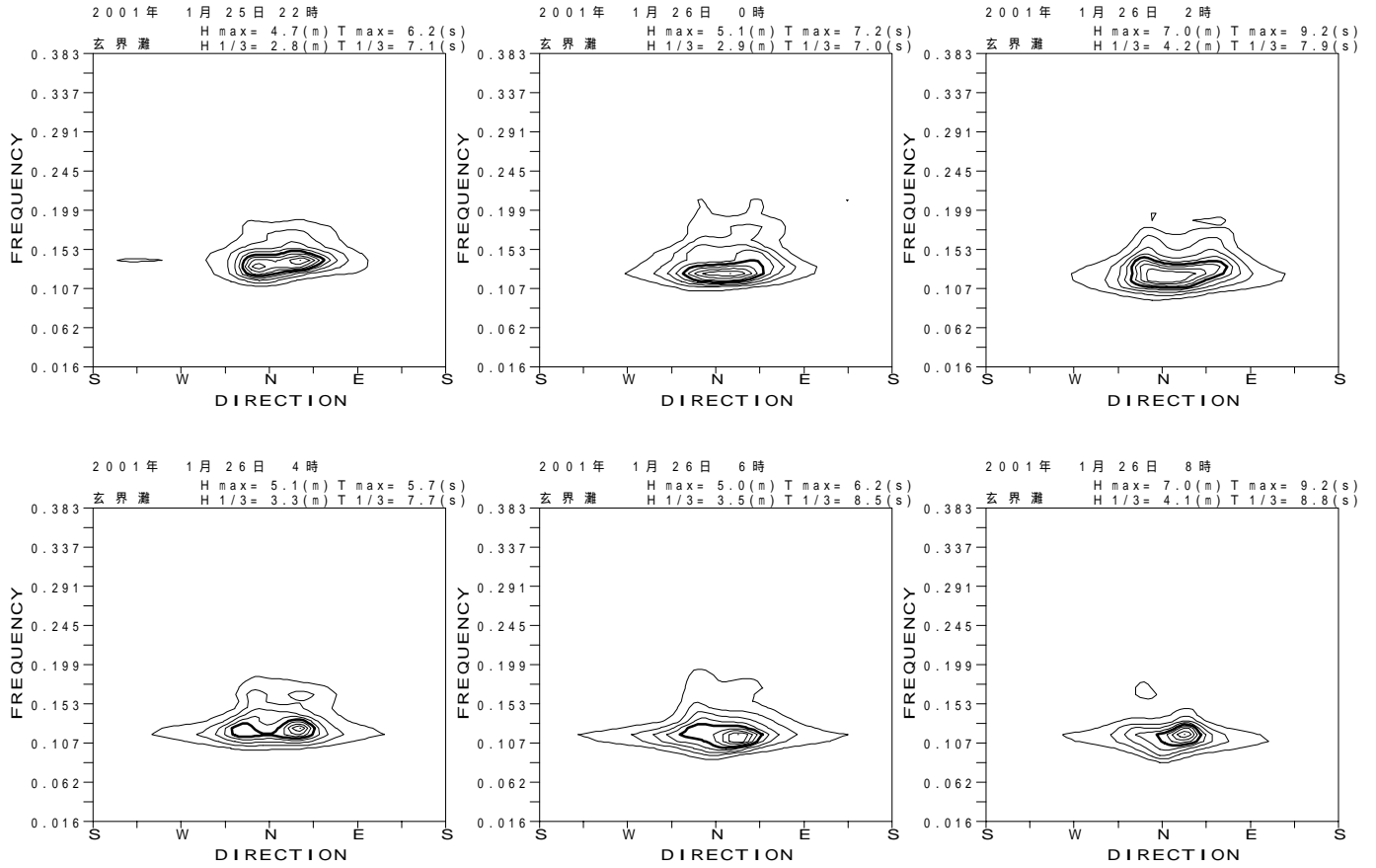
付図 - B.3.17 玄界灘 代表的な高波期間中の方向スペクトル
