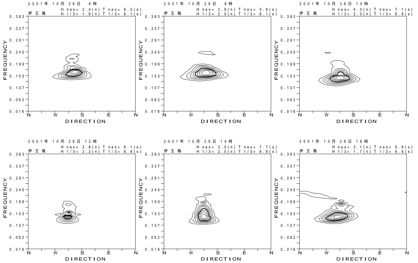
付図 - B.3.18 伊王島 代表的な高波期間中の方向スペクトル
