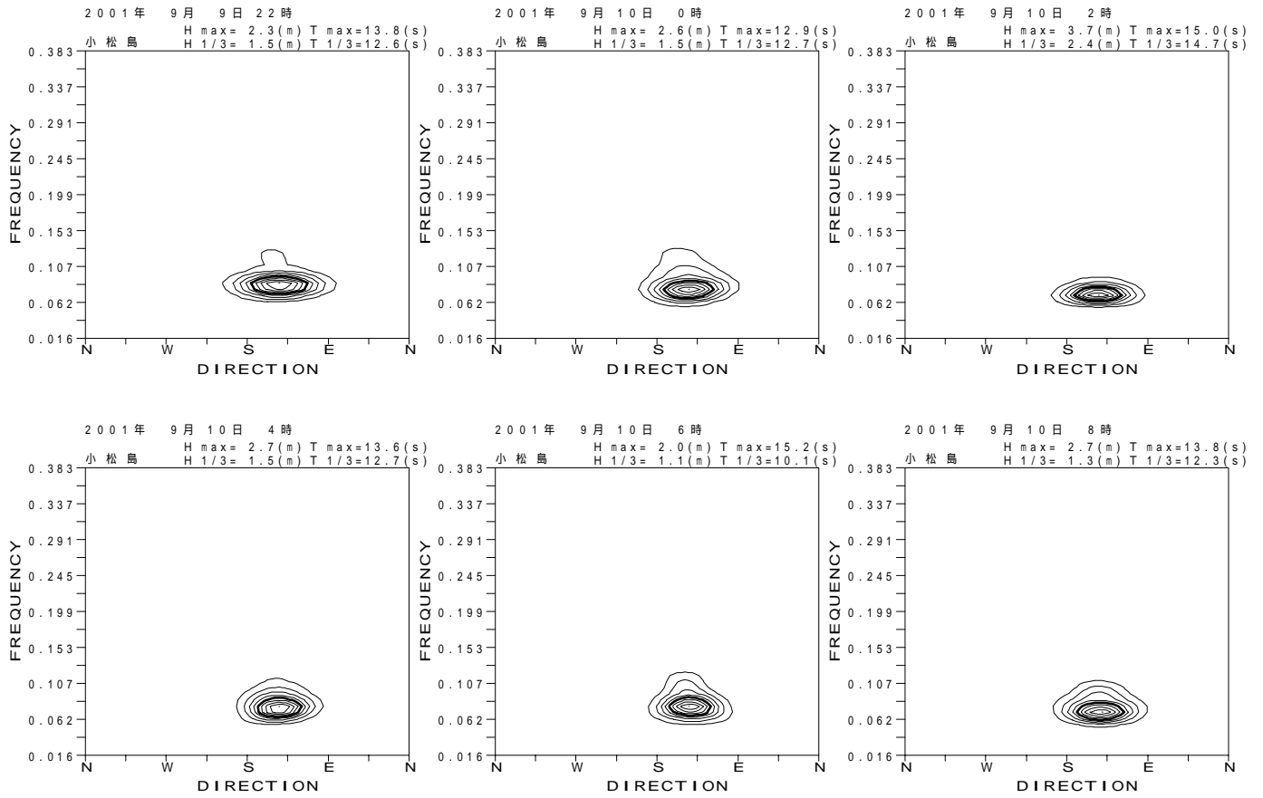
付図 - B.3.42 小松島 代表的な高波期間中の方向スペクトル
