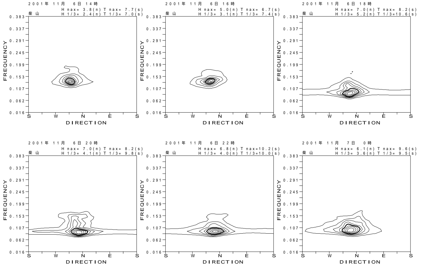
付図 - B.3.11 柴山 代表的な高波期間中の方向スペクトル
