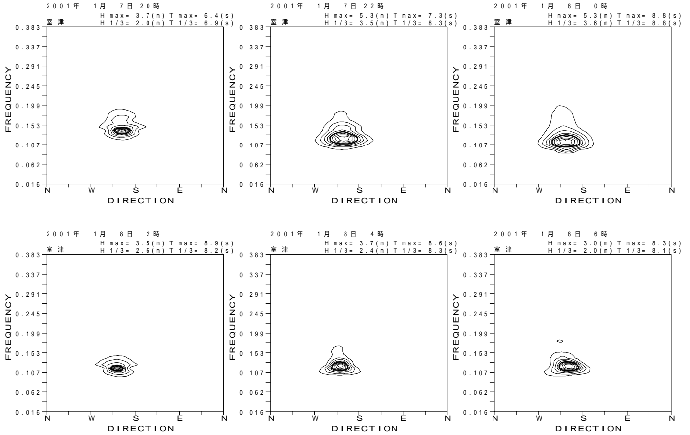
付図 - B.3.43 室津 代表的な高波期間中の方向スペクトル
