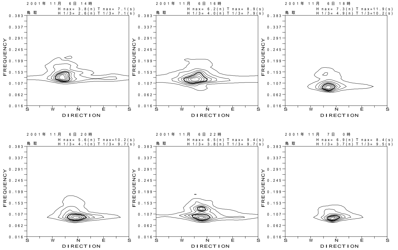
付図 - B.3.13 鳥取 代表的な高波期間中の方向スペクトル
