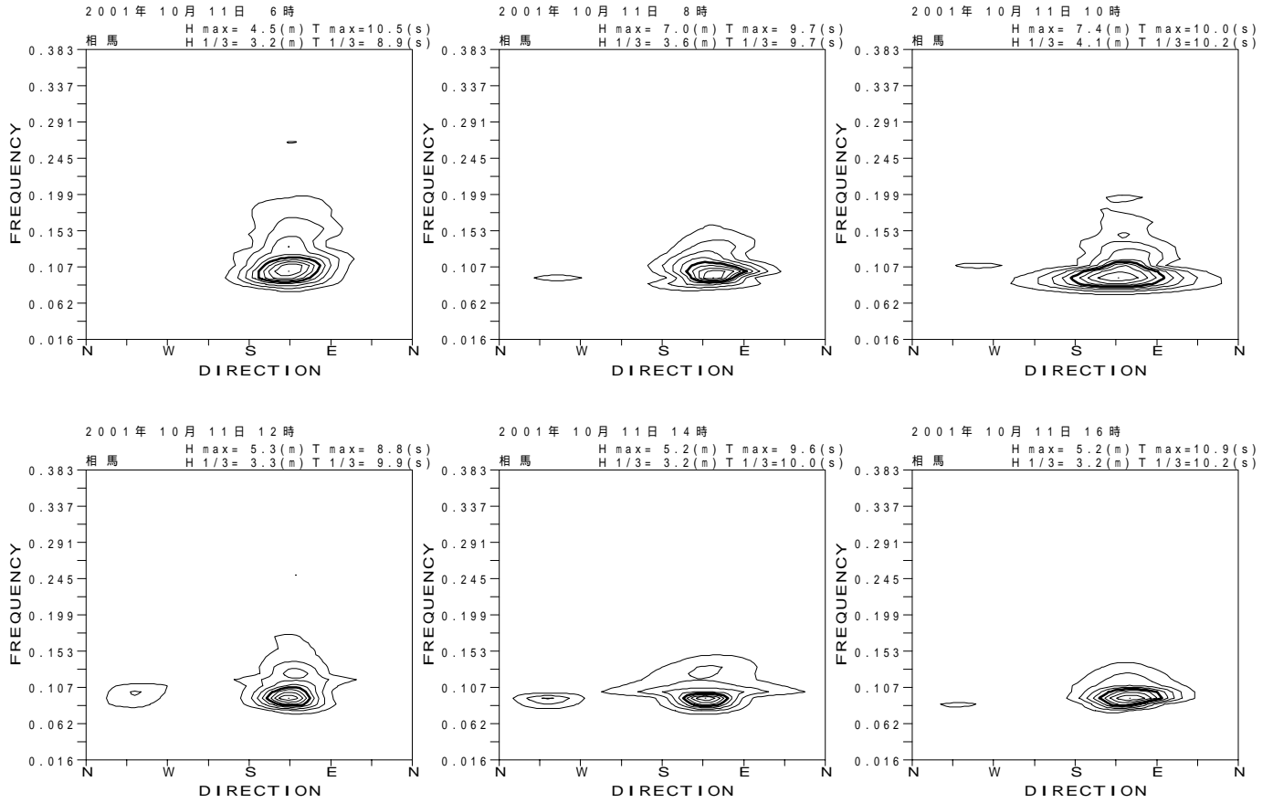
付図 - B.3.30 相馬 代表的な高波期間中の方向スペクトル
