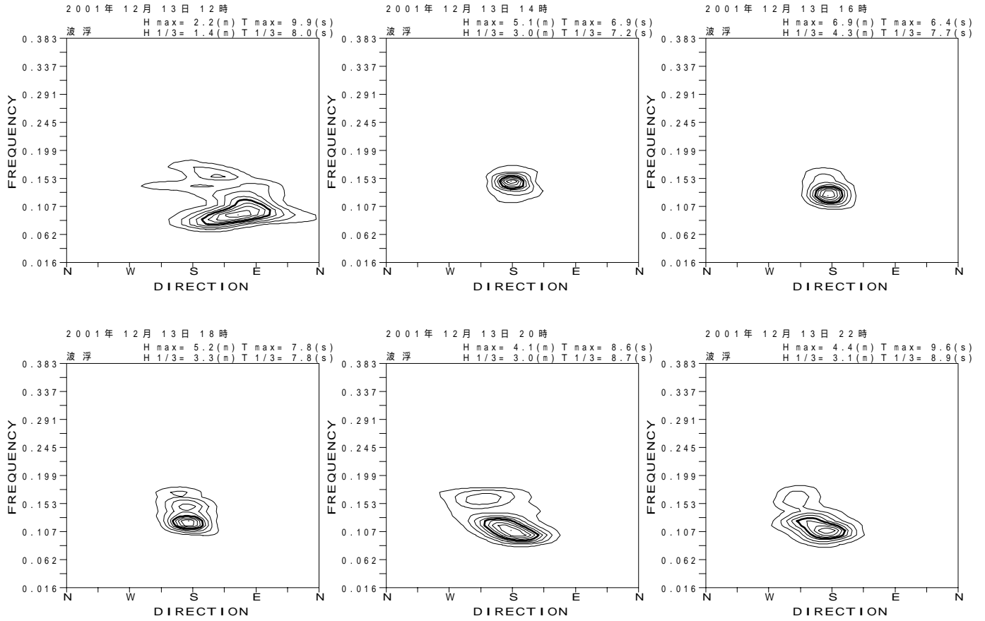
付図 - B.3.36 波浮 代表的な高波期間中の方向スペクトル
