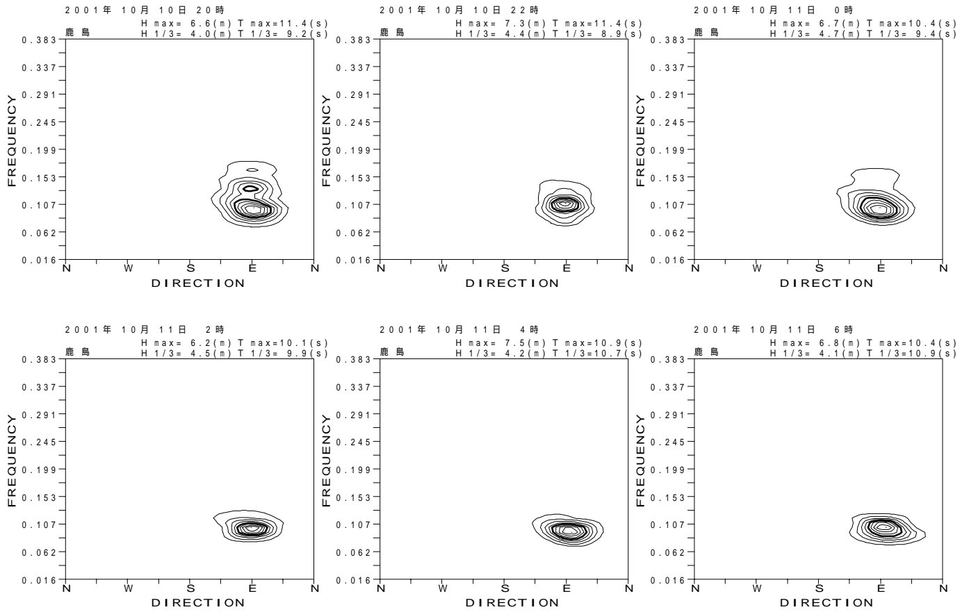
付図 - B.3.33 鹿島 代表的な高波期間中の方向スペクトル
