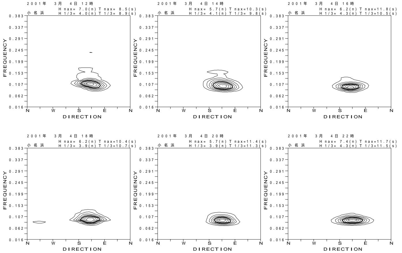
付図 - B.3.31 小名浜 代表的な高波期間中の方向スペクトル
