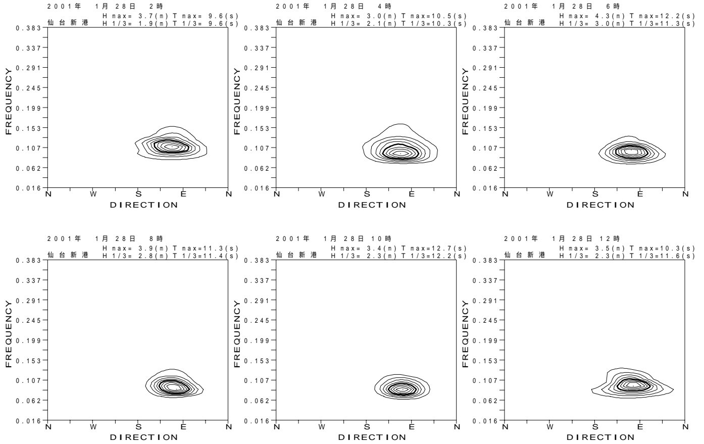
付図 - B.3.29 仙台新港 代表的な高波期間中の方向スペクトル
