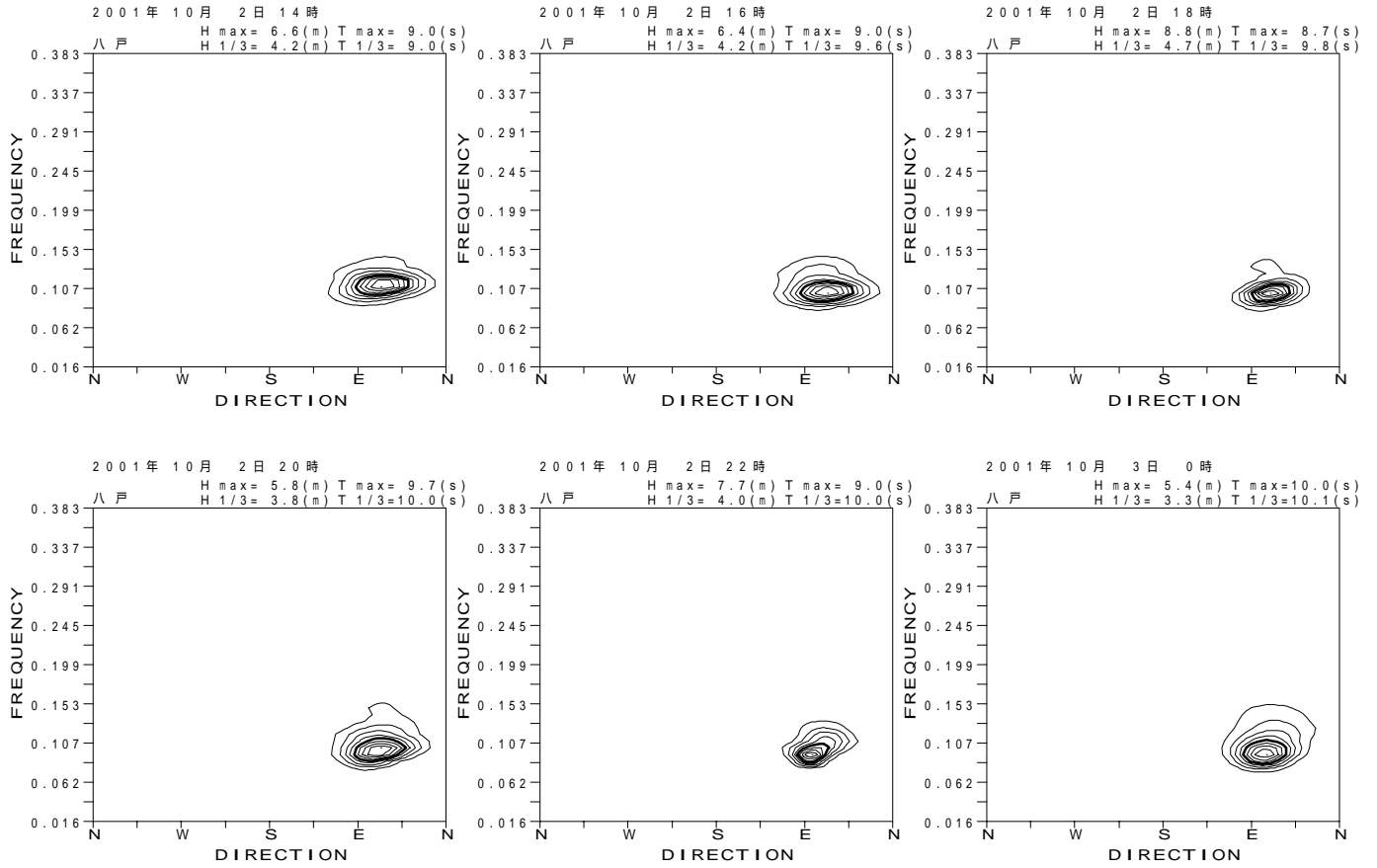
付図 - B.3.26 八戸 代表的な高波期間中の方向スペクトル
