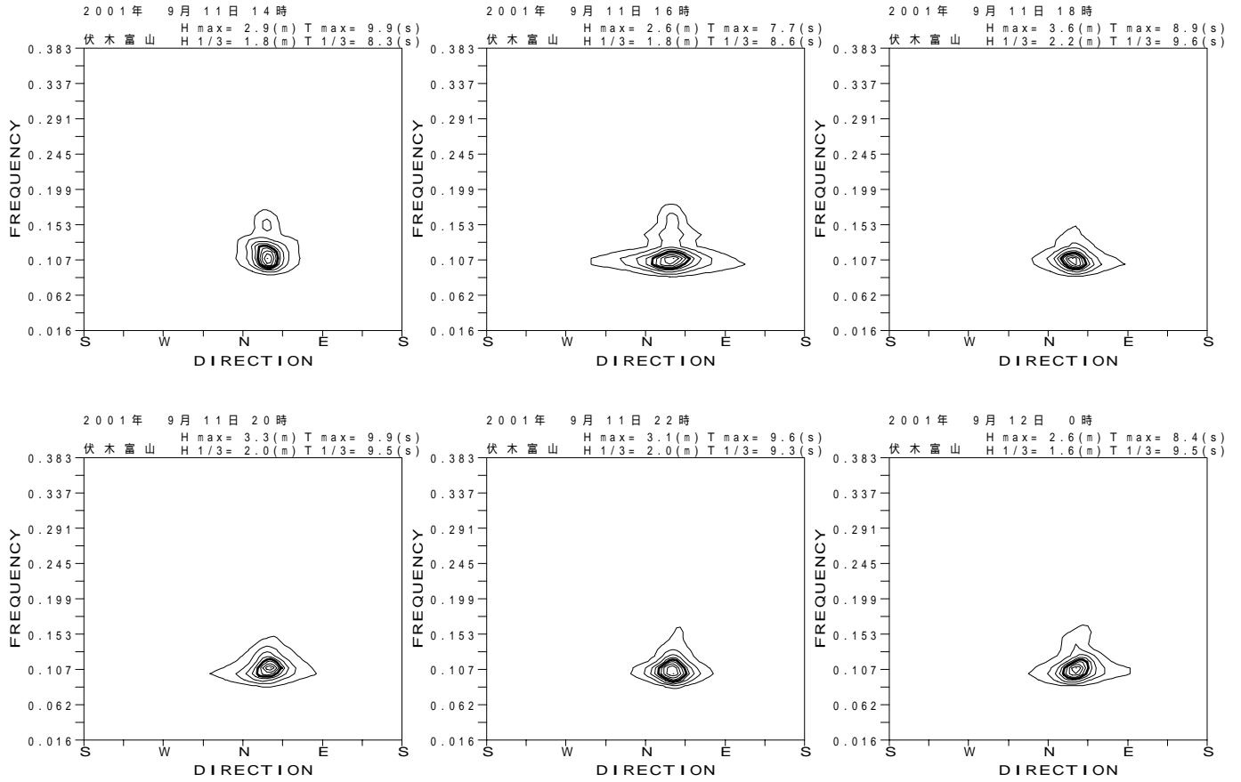
付図 - B.3.8 伏木富山 代表的な高波期間中の方向スペクトル
