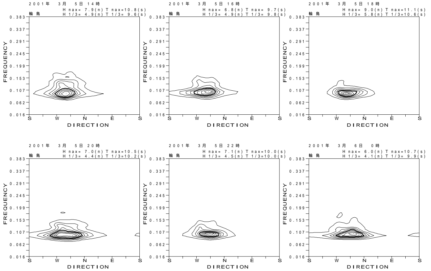
付図 - B.3.9 輪島 代表的な高波期間中の方向スペクトル
