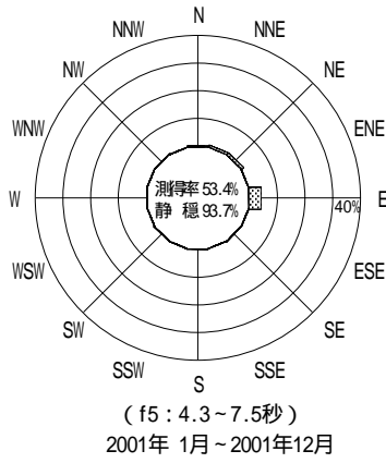
付図 - B.2.46 苅田 波高・波向別出現頻度図 ( f2 , f3 , f4 , f5 , 全周期帯 )
